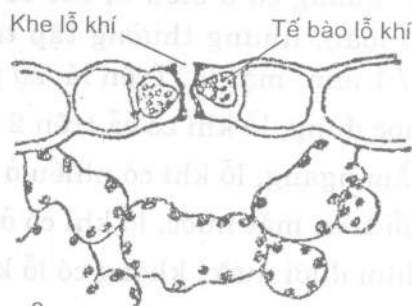
Hình 2.3. Biểu bì và lỗ khí
