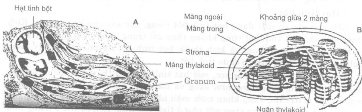
Hình 1.16. Cấu tạo của lục lạp
