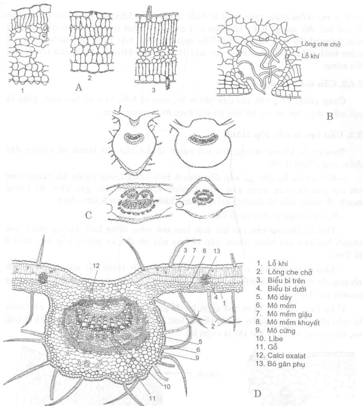
Hình 3.18. Các dạng cấu tạo thịt lá (A) (1: Dị thể bất đối xứng, 2: Đồng thể, 3: Dị thể đối xứng), phòng ảnh lỗ khí (B), các dạng cấu tạo gân lá lớp Ngọc lan (C) và cấu tạo vi học lá Ô môi ( Cassia grandis ) (D)
