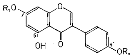
Genistin
